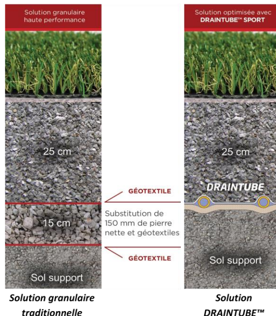
Comparaison entre une solution granulaire haute performance et la solution optimisée DRAINTUBE® pour le drainage de la fondation d'un terrain sportif.
