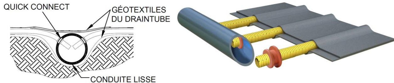
Figures 8: Système Quick Connect
