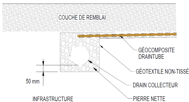
Figures 7: Raccordement à une tranchée collectrice
